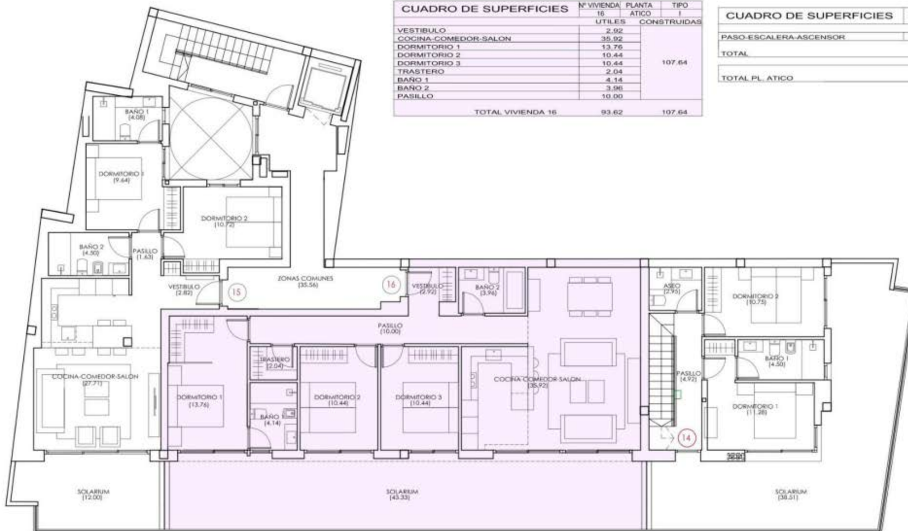
PLANTA ATICO 4
