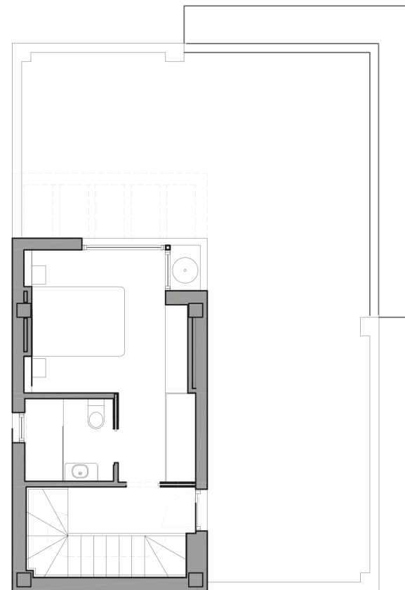
PLANTA PRIMERA
