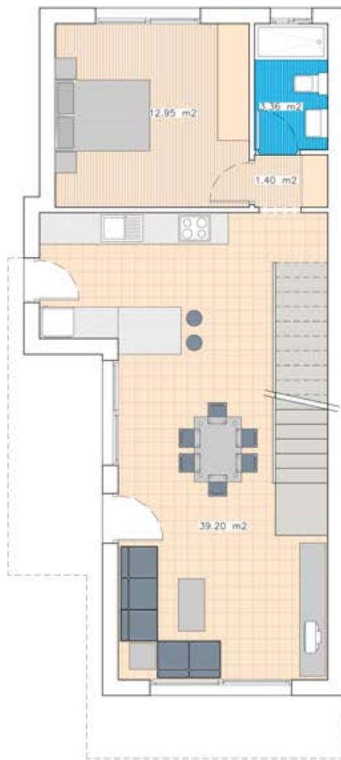
PLANTA BAJA
