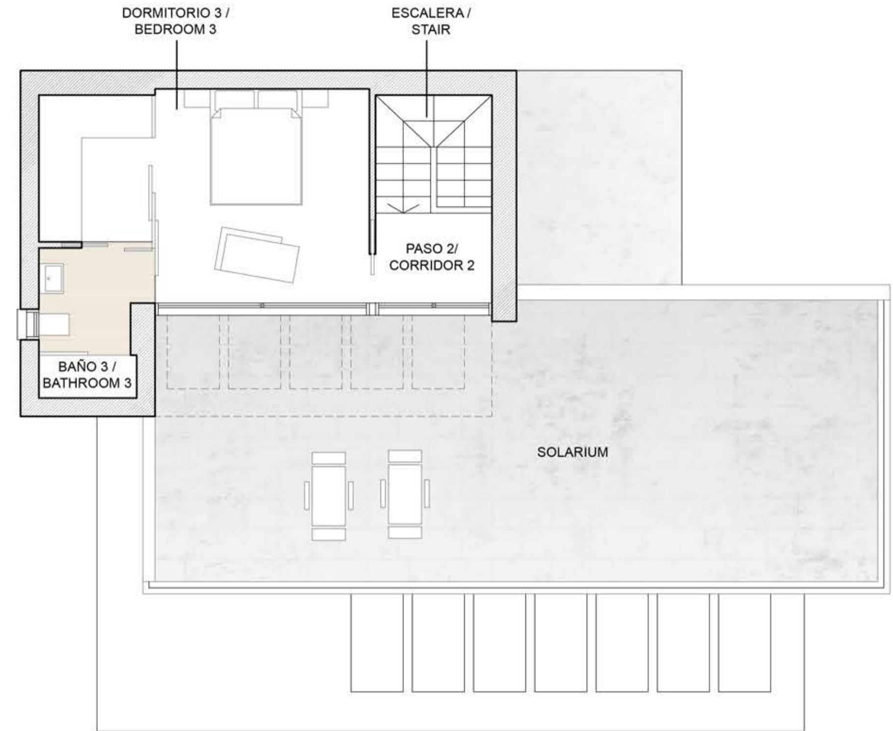
PLANTA ALTA / TOP FLOOR
