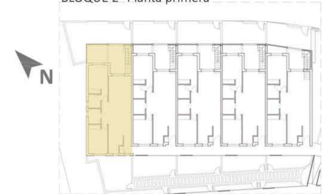
BLOQUE 2- Planta primera
